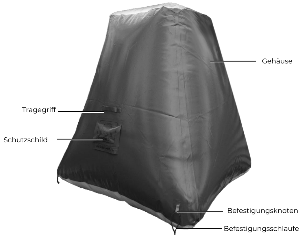
Die Hauptbestandteile des aufblasbaren Schutzes
